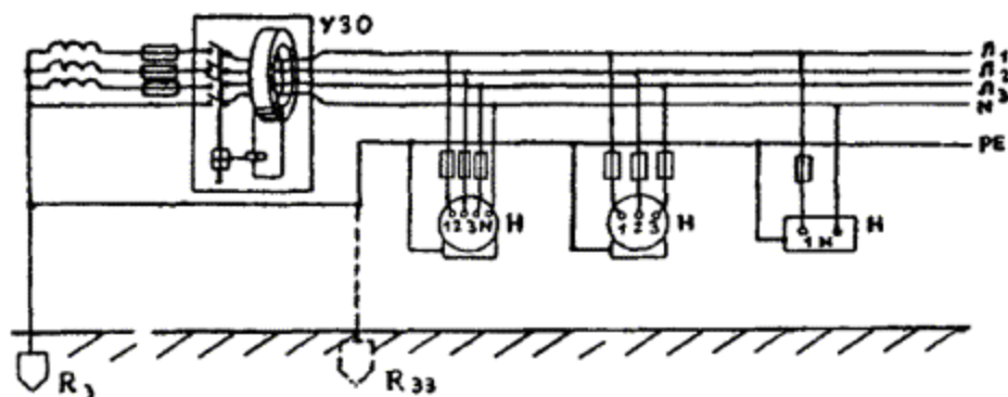
Рис. 2.2.7. Схема установки УЗО в четырехпроводной сети с глухозаземленной нейтралью в системе TN-S (нулевой рабочий N и нулевой защитный PE проводники разъединены):
