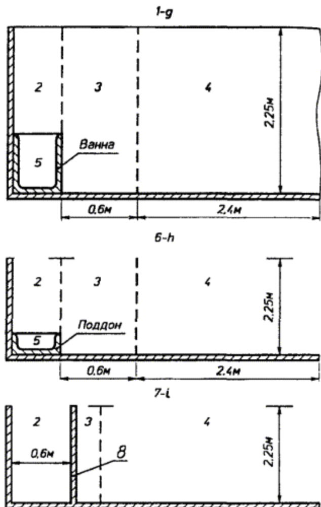
Рис. 2.2.9.б. Зоны в ванных и душевых помещениях, вертикальный разрез (согласно ГОСТ Р 50571.11-96 .):
