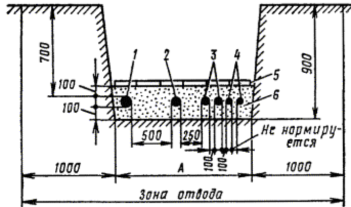
Рис. 3.2.3. Минимальные расстояния между кабелями, прокладываемыми в траншеях:
