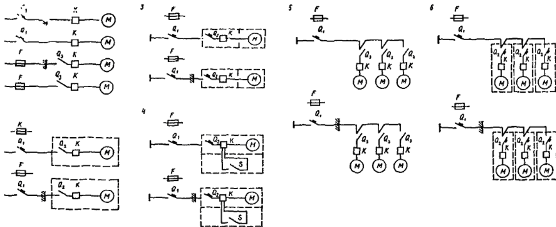
Рис. 2.4.1 (1-6). Схемы присоединения силовых электроприемников холодильного оборудования:
