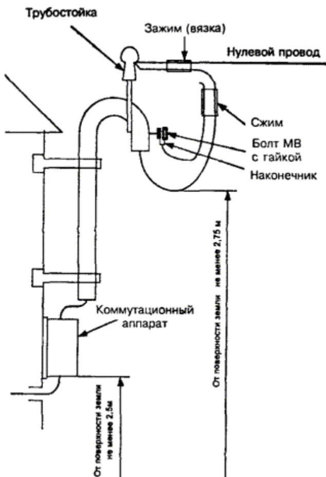
Рис. 2.3.3. Устройство ввода в здание через трубостойку.
