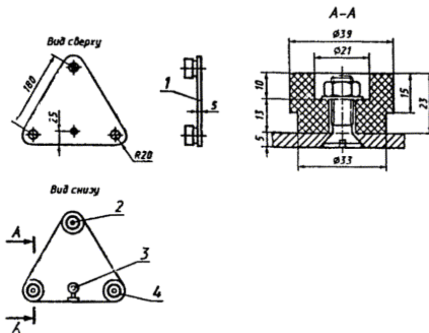
Рис. А.1. Испытательный электрод 2
