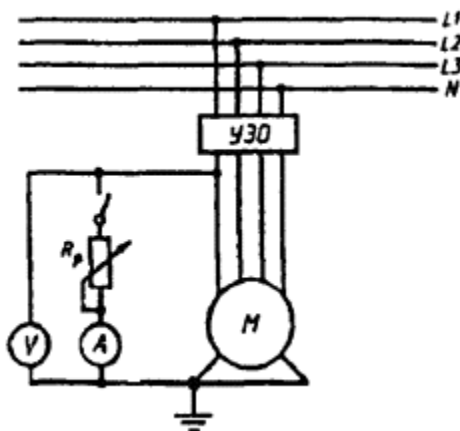
Рис. В.1. Схема проверки УЗО по методу 1.
