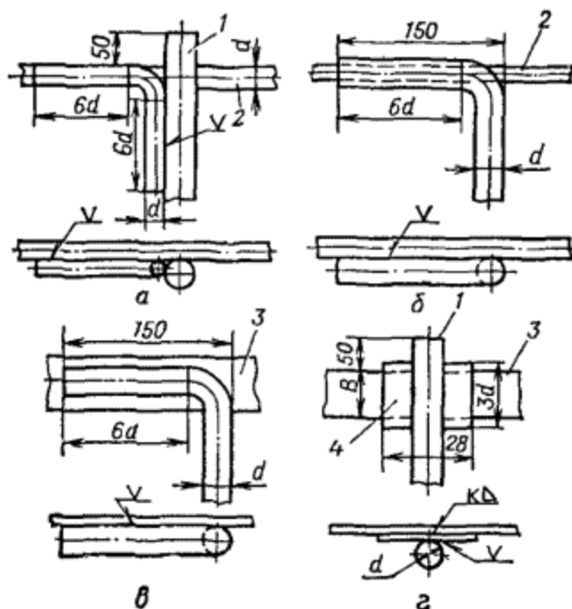
Рис. 3.1.1. Соединение стержневых электродов с заземляющими проводниками (длина сварного шва 6d ):
