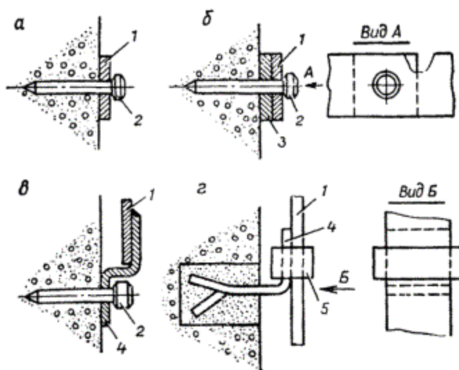
Рис. 3.1.4. Способы крепления заземляющих проводников из полосовой стали:
