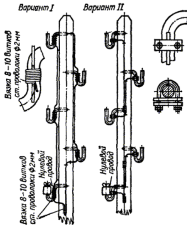
Рис. 3.3.4. Заземление крюков ВЛ 0,4 кВ на деревянных опорах.
