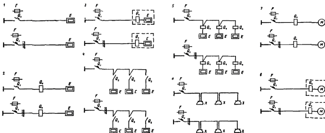
Рис. 2.4.2 (1-8). Схемы присоединения силовых электроприемников технологического (теплового или механического) оборудования:
