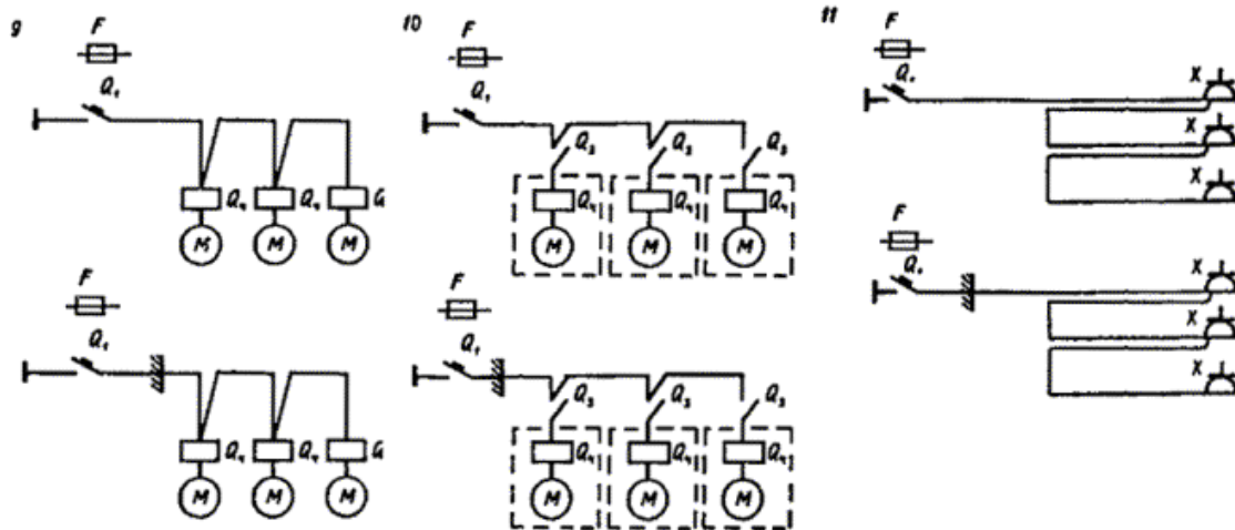
Рис. 2.4.2 (9-11). Схемы присоединения силовых электроприемников технологического (теплового или механического) оборудования:
