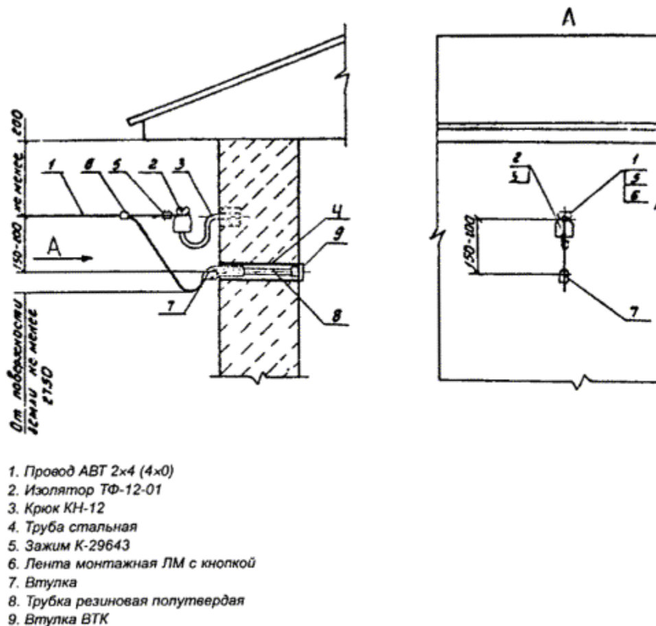
Рис. 2.2.3. Устройство воздушного ввода от ВЛ тросовым проводом. Стены кирпичные (бетонные).
