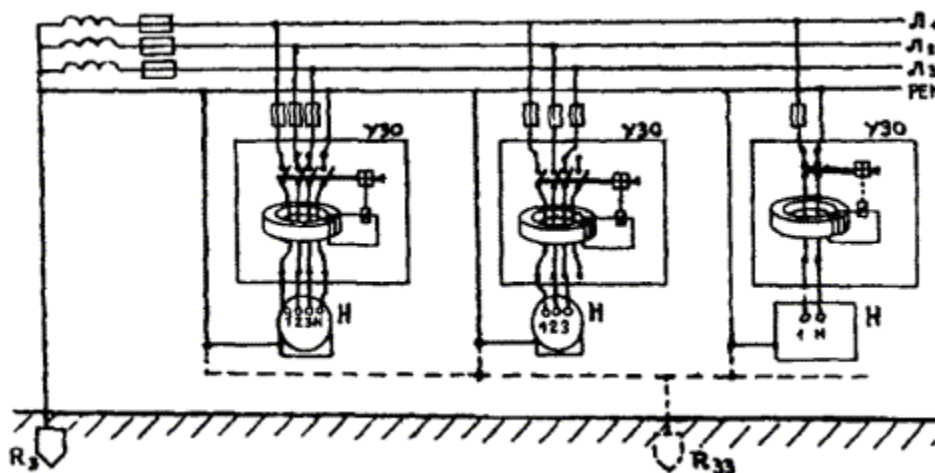
Рис. 2.2.6. Схема установки УЗО в четырехпроводной сети с глухозаземленной нейтралью в системе TN-C (нулевой рабочий N и нулевой защитный PE проводники объединены):
