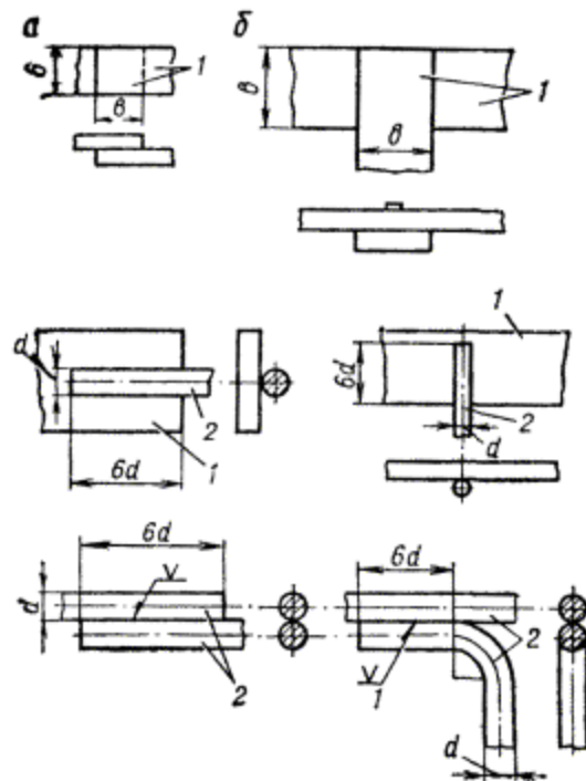
Рис. 3.1.5. Сварные соединения заземляющих проводников:
