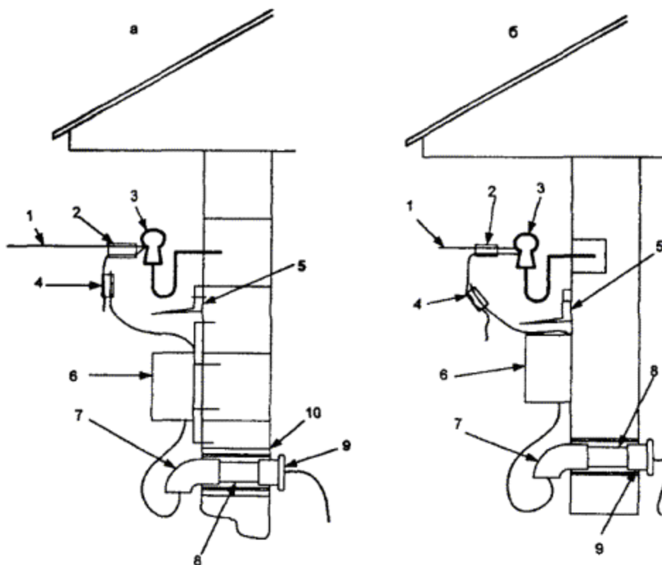
Рис. 2.3.2. Устройство ввода в здание:
