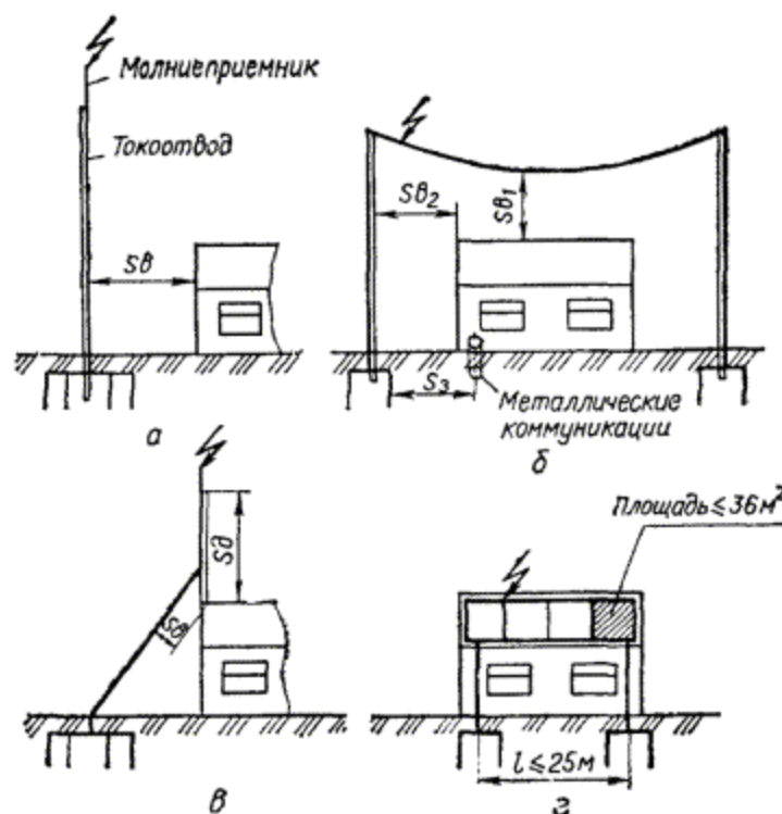
Рис. 3.4.1. Типы молниеотводов:
