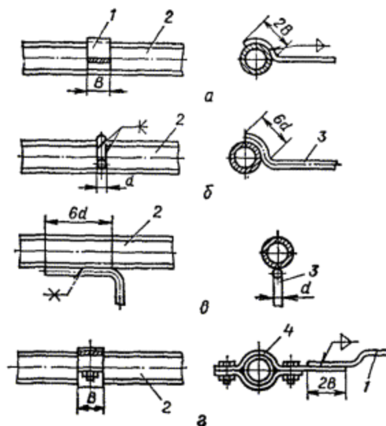
Рис. 3.1.2. Примеры присоединения заземляющих проводников к трубопроводам:
