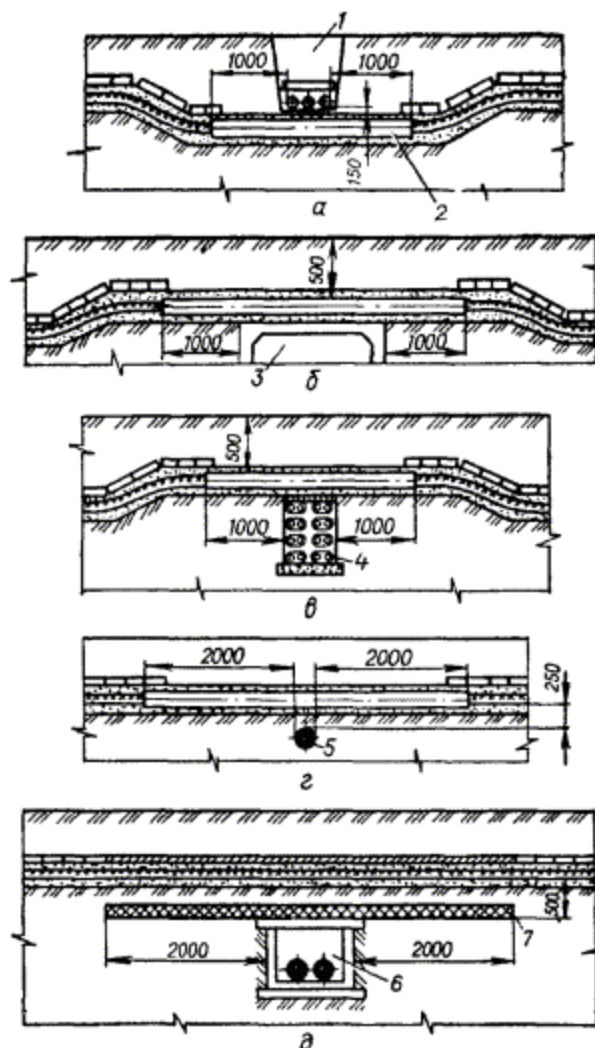
Рис. 3.2.1. Пересечение кабельных траншей с другими коммуникациями:
