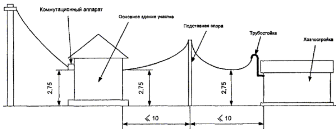
Рис. 2.3.1. Внутриобъектная электропроводка (размеры даны в метрах).
