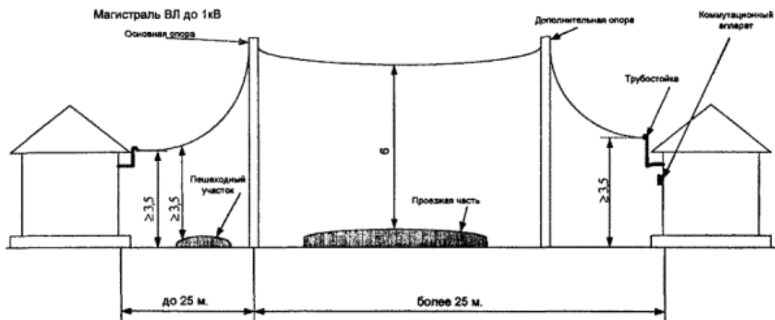
Рис. 2.2.1. Расстояние от проводов ВЛ до 1 кВ при наибольшей стреле провеса до земли, проезжей части улицы, тротуаров или пешеходных дорожек.
