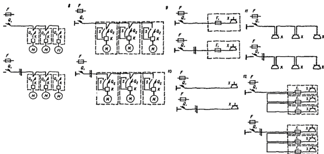
Рис. 2.4.1 (7-12). Схемы присоединения силовых электроприемников холодильного оборудования:
