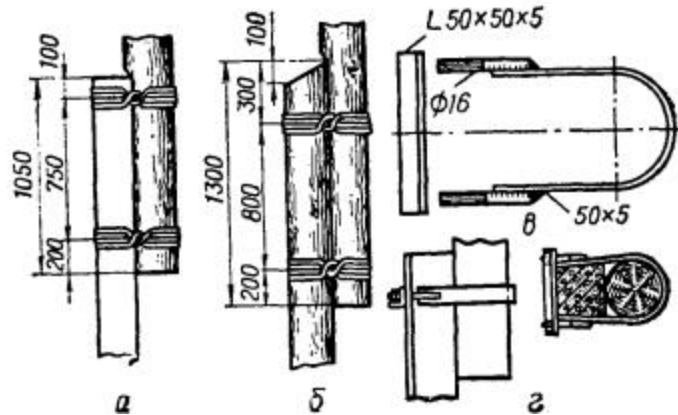
Рис. 3.3.3. Соединение стойки опор ВЛ 0,4 кВ с приставкой:
