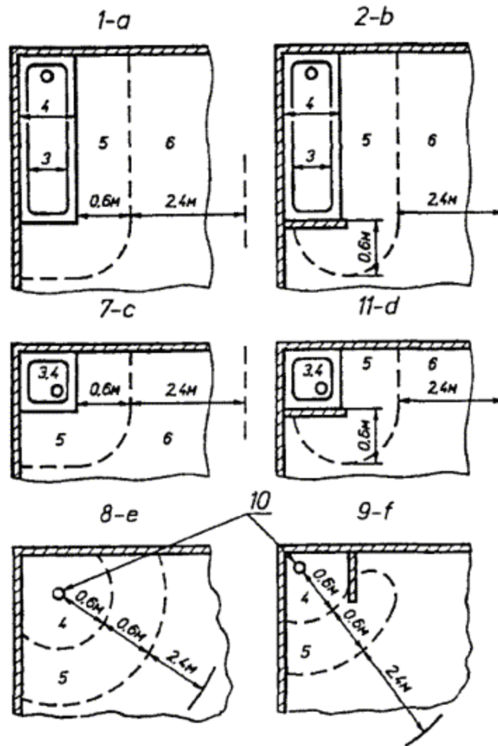
Рис. 2.2.9.а. Зоны в ваннах и душевых помещениях, план (согласно ГОСТ Р-50571.11-96. ):
