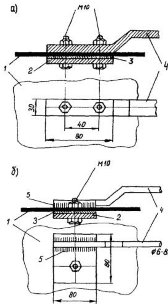
Рис. 3.4.3. Зажим для присоединения плоского (а) и круглого (б) токоотводов к металлической кровле:
