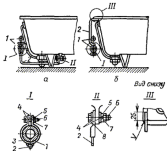
Рис. 3.1.6. Заземления корпуса ванны:
