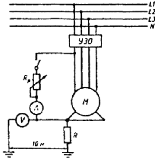
Рис. В.3. Схема проверки УЗО по методу 3.
